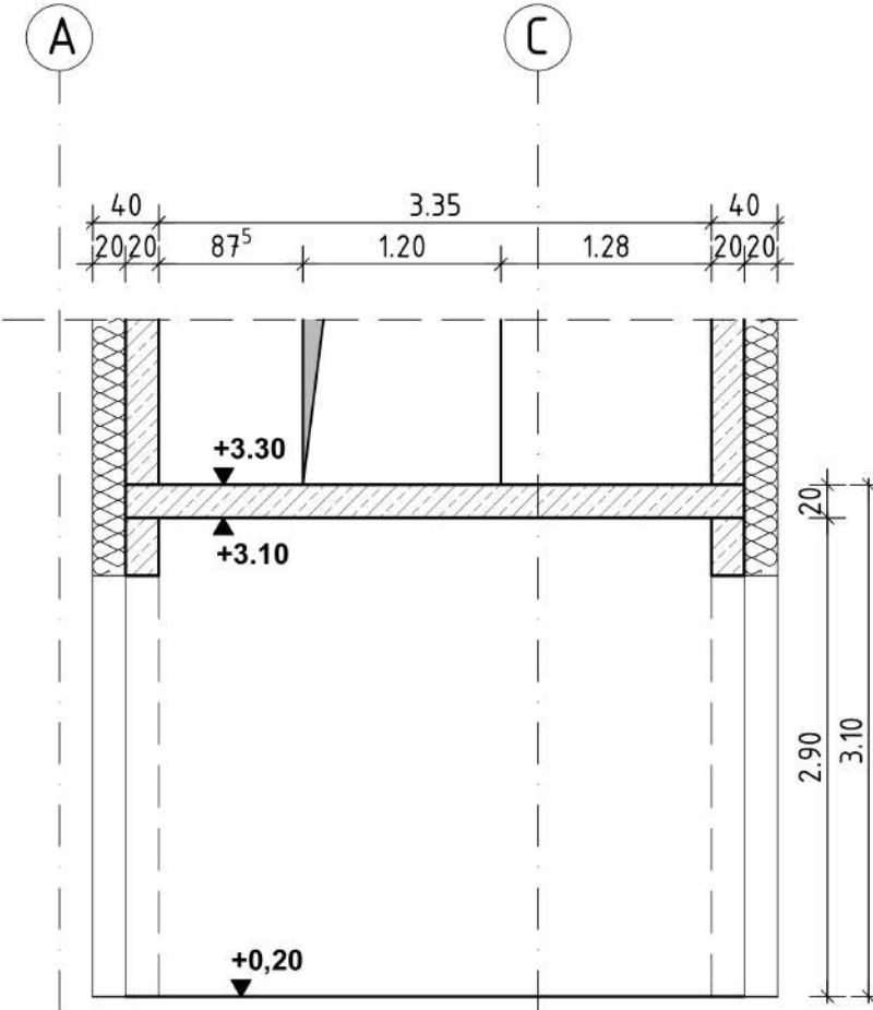
Schnitt 3-3 M 1:50
