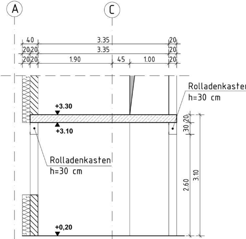
Schnitt 4-4 M 1:50
