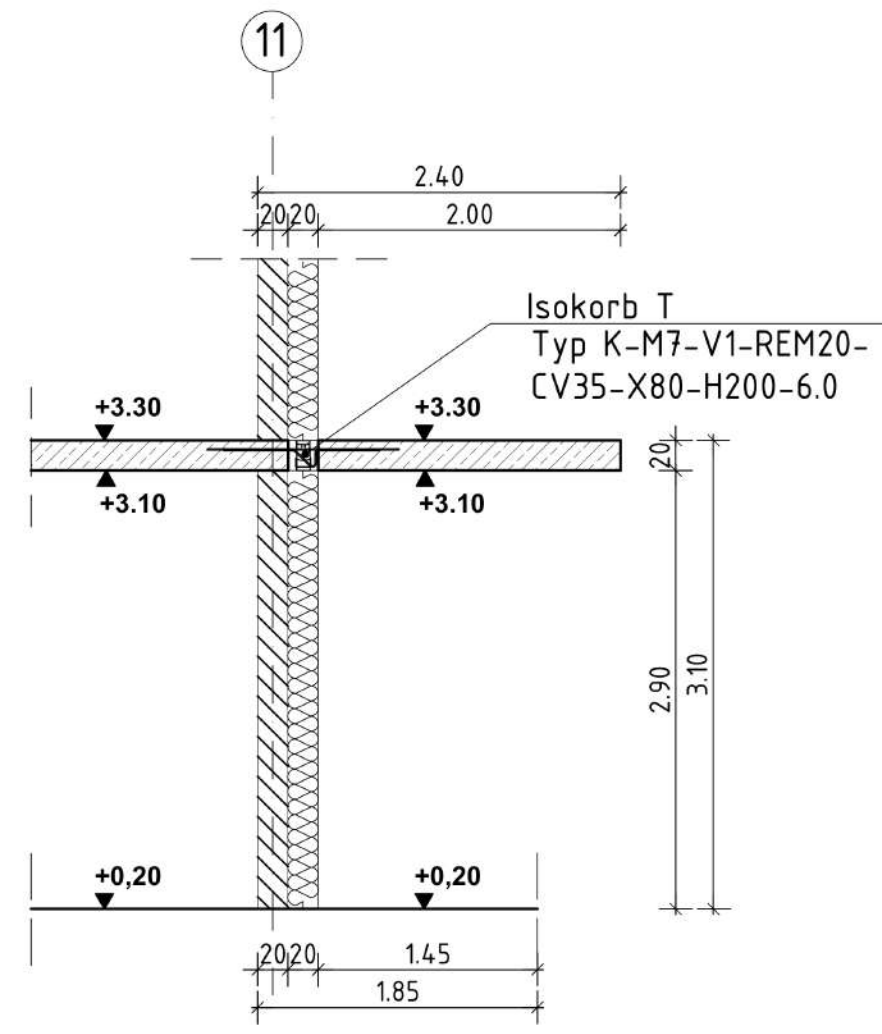
Schnitt 1-1 M 1:50
