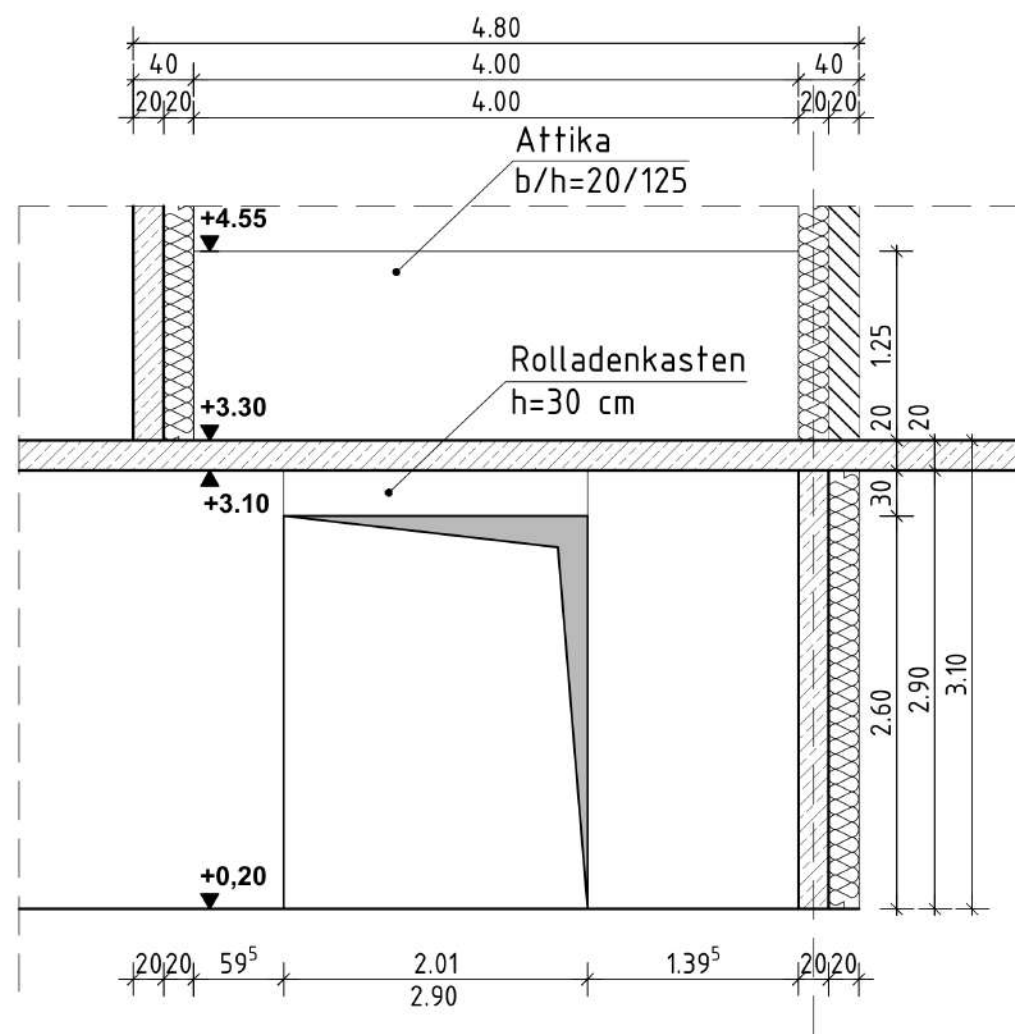
Schnitt 5-5 M 1:50
