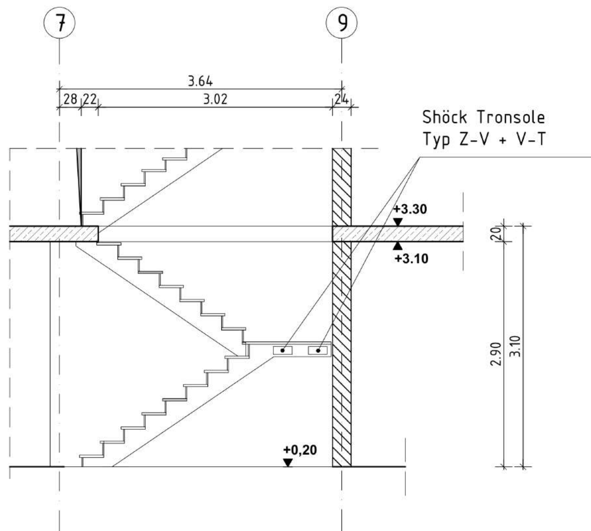
Schnitt 2-2 M 1:50
